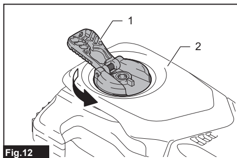
Fig.12 ► 1. Palanca 2. Cubierta de la pieza dentada
