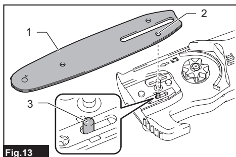
Fig.13 ► 1. Barra de guía 2. Orificio 3. Pasador
