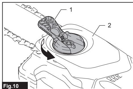
Fig.10 ► 1. Palanca 2. Cubierta de la pieza dentada
